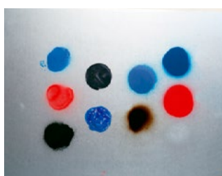
Przed oraz po 15 cyklach graffiti i czyszczenia
